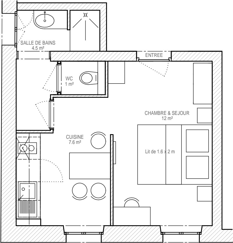
Implantation appartements SEPPI & FRANTZ
